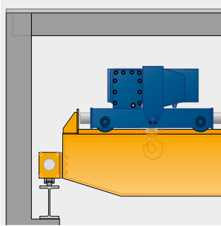
Aufgebockte Ausführung Variante 2
