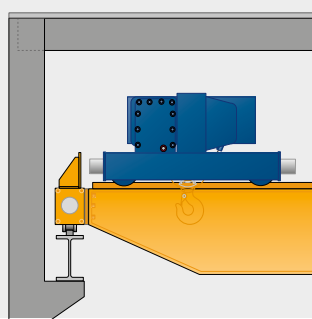
Serienhauptträger-Anschluss Variante 1
