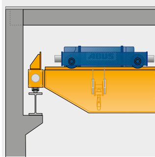
Serienhauptträger-Anschluss Variante 1 in Kombination mit abgesenkter Katze
